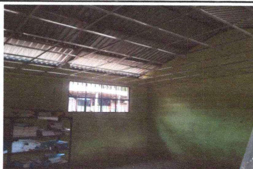
Foto 6: Instalacion de Base de Cielo Falso.
