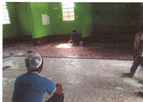
Foto 2: Colocacion de Piso Ceramico.
